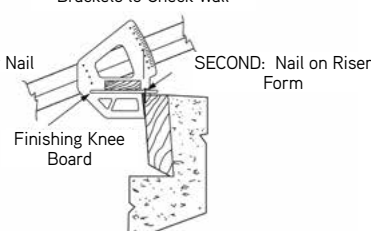
Battered Riser
