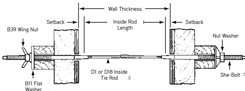
D2, D30 She-Bolt
